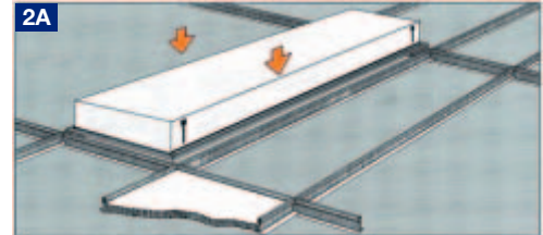
2A Instalación en techo perfil visto. Luminaire installed in a T-bar ceiling.
