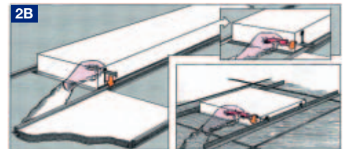
2B Instalación mediante uso de garras. Luminaire instaled using brackets.
